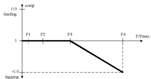
圖 1 智慧變流器 \cos\phi(P) 曲線
